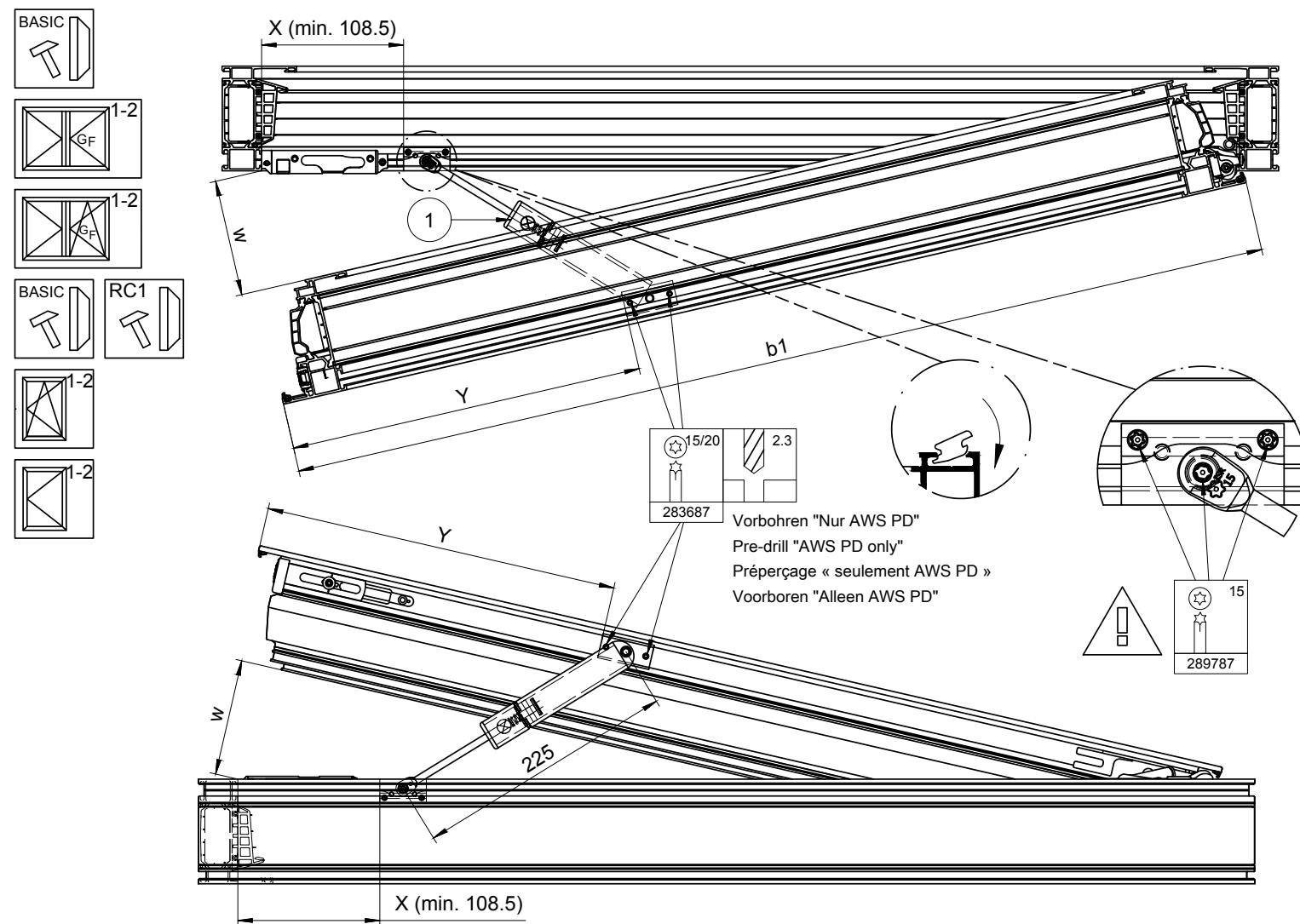
Ansicht von unten View from below Vue de dessous Onderaanzicht
