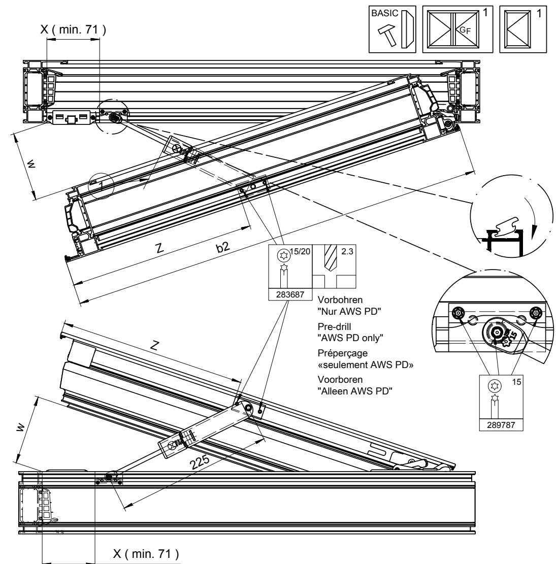
Ansicht von unten View from below Vue de dessous Onderaanzicht
